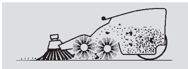
Doppelwalzensystem und Seitenbesen
